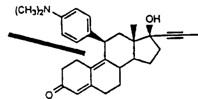
RU 486
